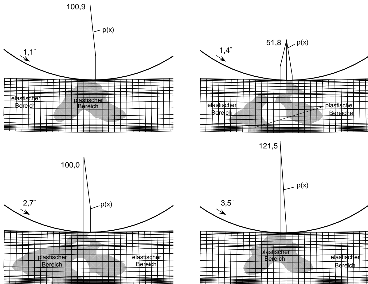
Abb. 7.28: Materialbeanspruchung und Kontaktpressung p(x) in kN/mm^2 während des Rollenrichtvorgangs in verschiedenen Rollinkrementen
