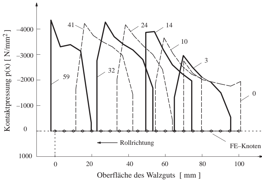
Abb. 7.32: Verteilung der Rollpressung in verschiedenen Walzsritten, \mu = 0,15
