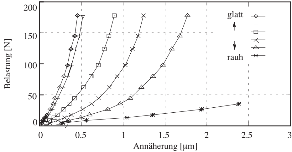
Abb. 4.1: Annäherung von Stahlflächen mit unterschiedlicher Rauigkeit im Normalkontakt (Nuri/Halling [86])
