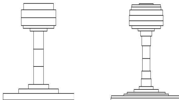
Abb. 7.11: Modellierung des Schienenprofils UIC 60 durch die Elementschichtung
