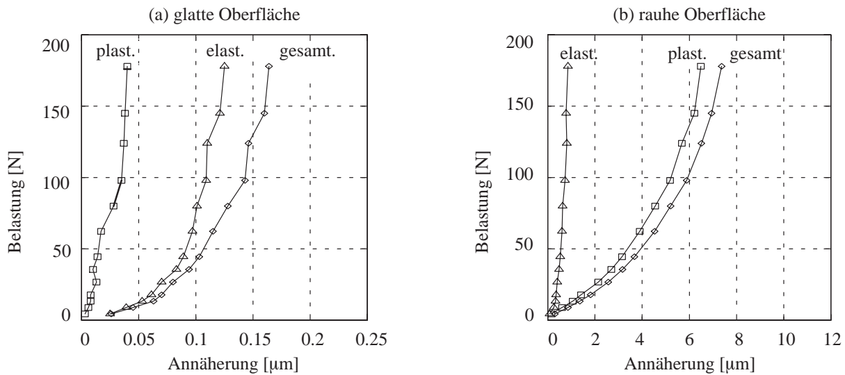
Abb. 4.2: Elastische und plastische Anteile bei der Annäherung von Stahlflächen (Nuri/Halling [86])
