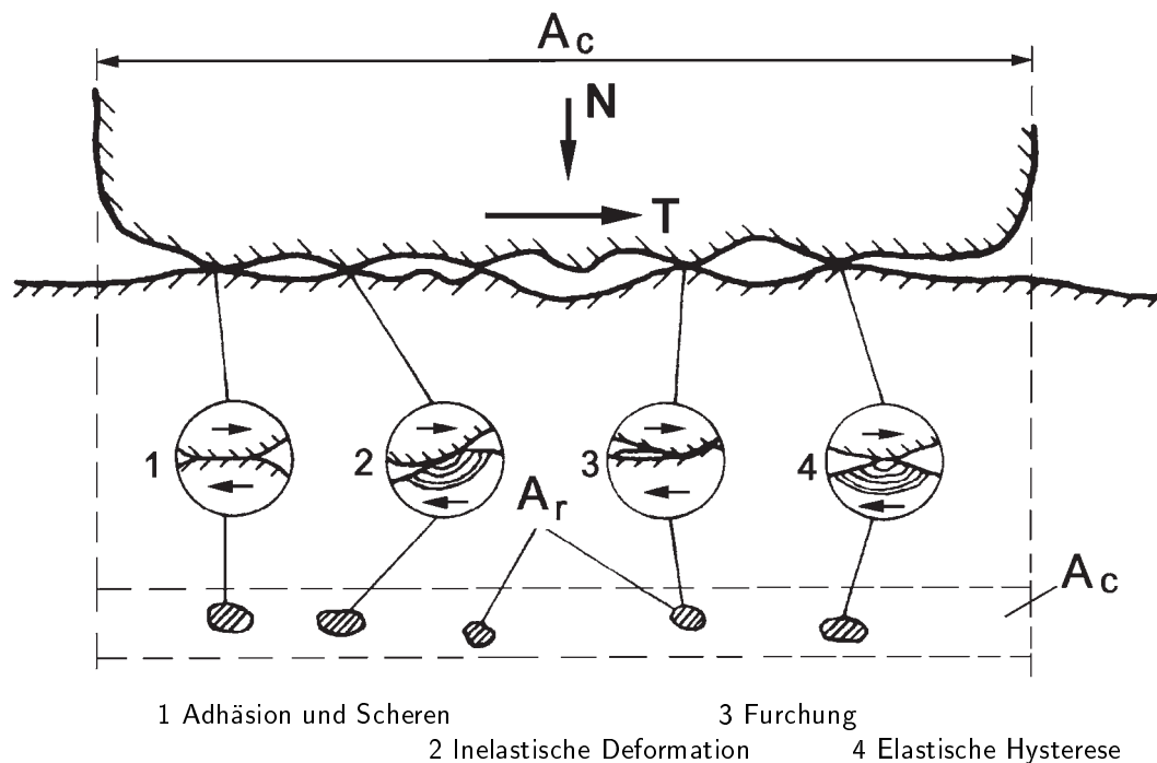
Abb. 2.4: Kontaktlokalisierung und Triboprozesse infolge der realen Oberflächenstruktur
