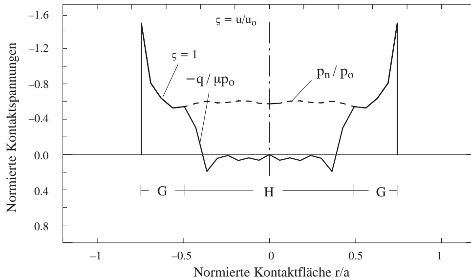
Abb. 7.7: Verteilung der Haft- und Gleitzonen in der Kontaktfläche mit maximalen Kontaktspannungen bei elasto-plastischem Materialverhalten
