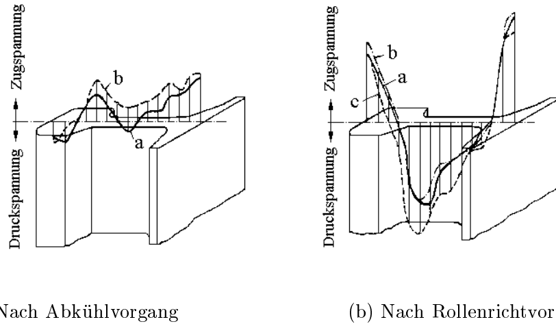
Abb. 1.5: Charakteristischer Eigenspannungsverlauf nach dem Abkühlvorgang (a-im Schienenstapel, b-allein liegend, c-spannungsarm gegläht) und nach dem Rollenrichtvorgang ( Meier [80])
