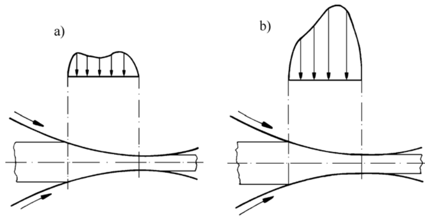
Abb. 1.3: Kontaktspannung beim Kaltwalzen von Stabstahl (a) und Bandstahl (b) (MacGregor/Palme [78], Malinowski/Lenard [79])
