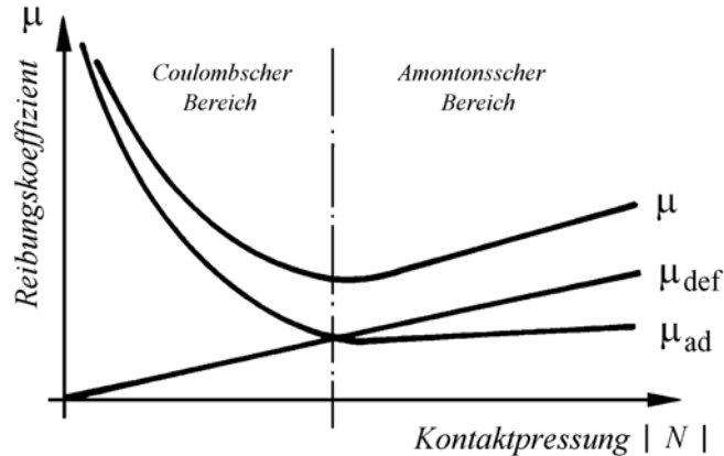
Abb. 2.5: Abhängigkeit des Reibwerts von der Normalbelastung ( Polzer/Meissner [91])
