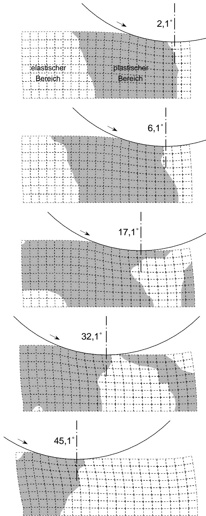
Abb. 7.35: Plastische Materialzonen im Walzgut unter fortschreitender Walzenrotation
