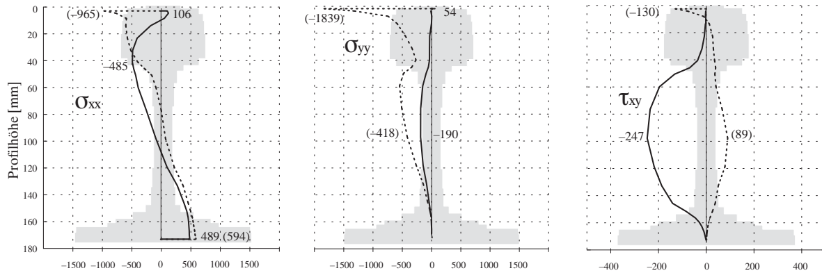
Abb. 7.25: Verteilung der Spannungskomponenten über die Schienenhöhe während (···) und nach (—) der Rollbelastung
